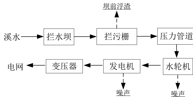
图 2.2.6-1 工程运行方式图
